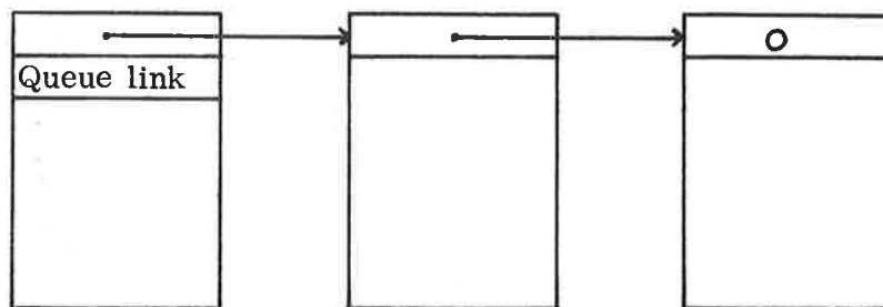
Fig. 4.1.2. Extended buffer
