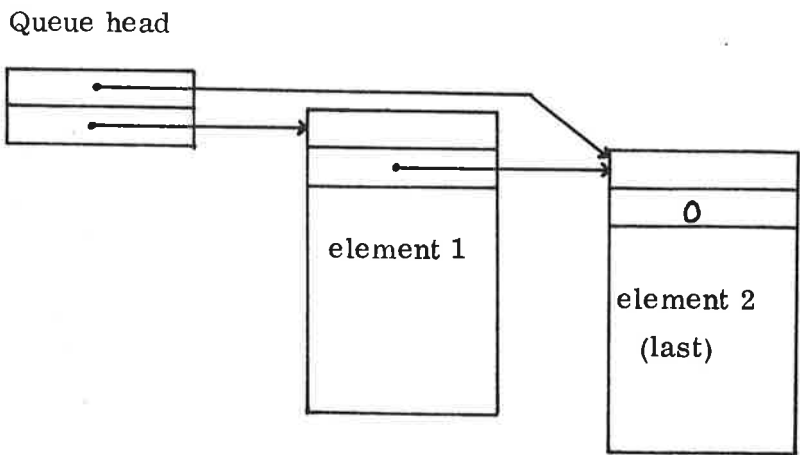
Fig. 4.1.1. Queue structure.
