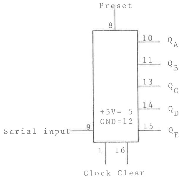
7496 5-bit shift register
