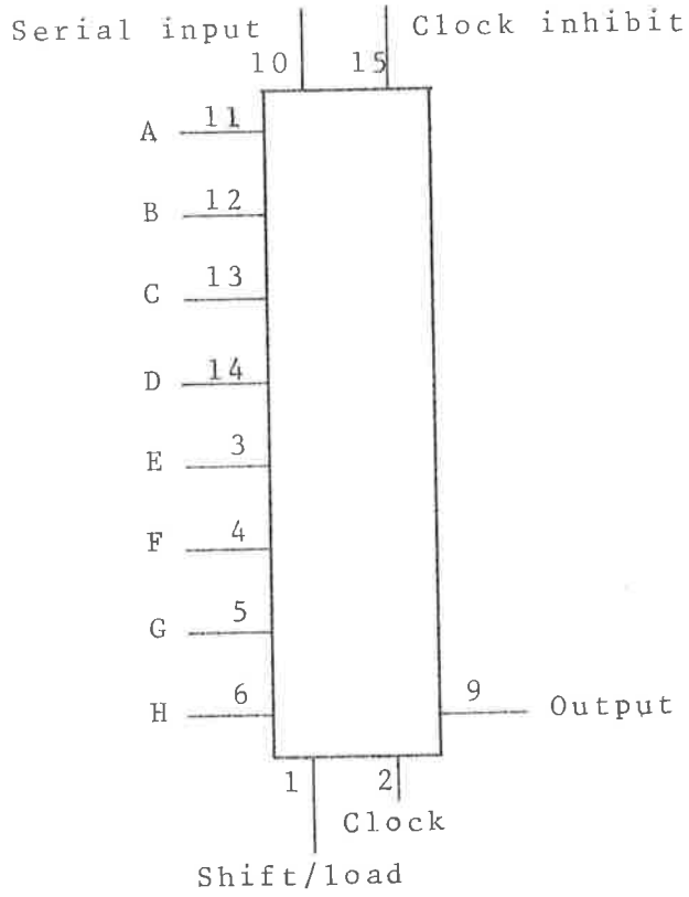
74165 8-bit shift register
